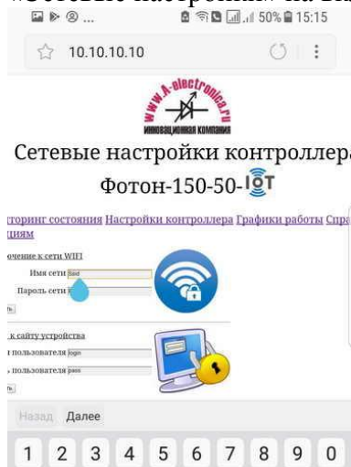
Рис.№3. Установка имени и пароля сети на сайте контроллера.
